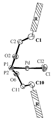
A) "RSSR"; ( 9a–e )
